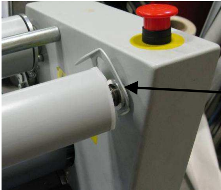
Figure 11 : Dispositif de verrouillage en haut
