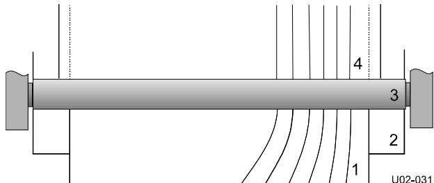
Abbildung 24: Falten aufgrund einer fehlerhaften Walzenausrichtung.
